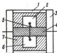
Рис. 1. Схема ввода дифференциальной термопары в камеру высокого давления. 1 — тальковая крышка; 2 — металлический висмут; 3 — тальковый изолирующий экран; 4 — тefлоновая или тальковая шайба; 5 — дифференциальная хромель-алюмелевая термопара; 6 — исследуемое вещество; 7 — передающая давление среда
